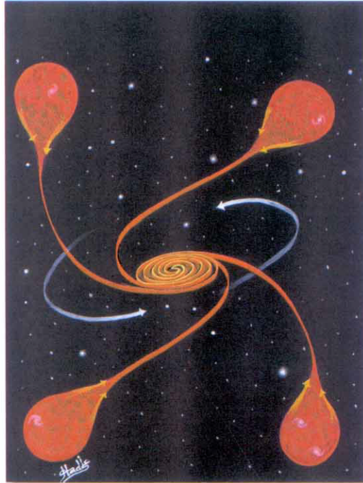
الثقب الأسود النهائي كما تبينه بعض الصور التوضيحية.
